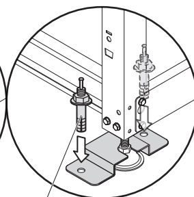
オールアンカー M10 (市販品) ※ 2ヶ所 / 本
