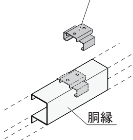
胴縁固定金具取付ネジ板
