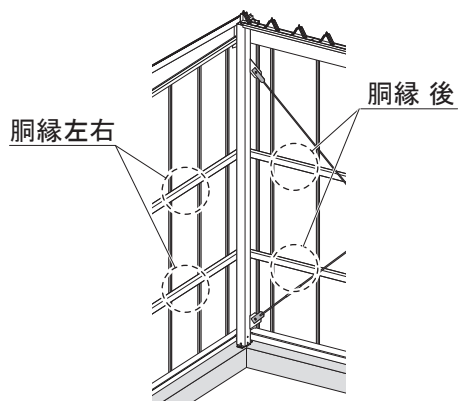
胴縁固定金具取付ネジ板
