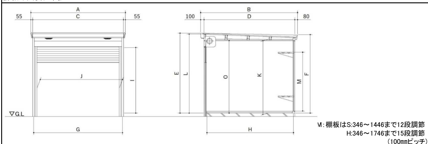
詳細寸法表(土間)
