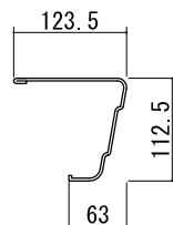
鼻隠し後 t=0.7
