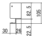
妻板固定金具 t=1.0
