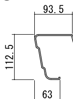
鼻隠し前 t=0.7
