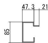
母屋 t=1.6
