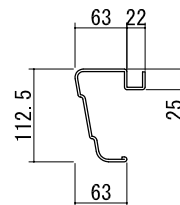
妻板 t=0.7
