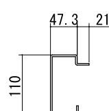
母屋 t=2.3
