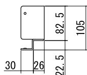
妻板固定金具 t=1.0
