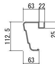
妻板 t=0.7
