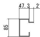
母屋 t=1.6
