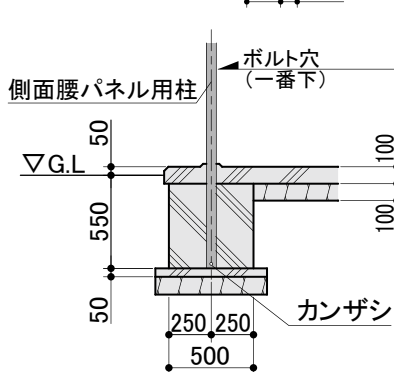
A-A' 断面 (S=1/40)
