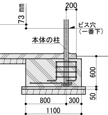
B-B' 断面 (例図: 埋め込み式)
