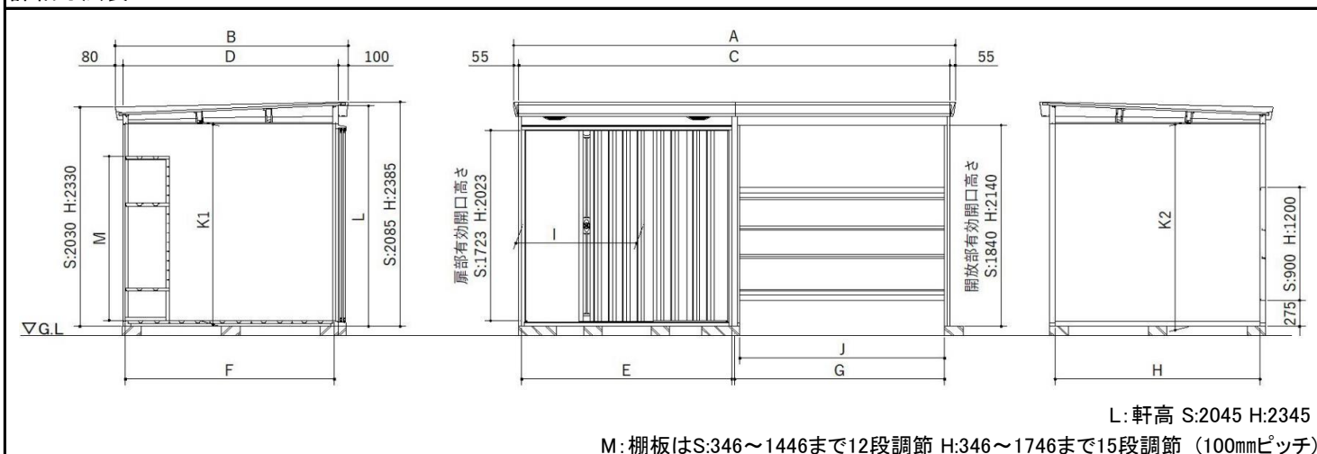
詳細寸法表
