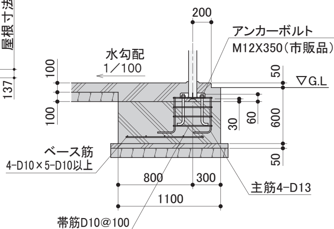
B-B' 断面 (S=1/40)
