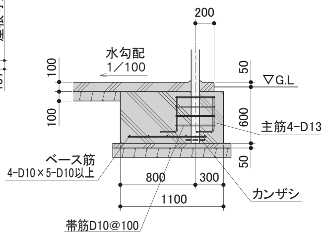
A-A' 断面 (S=1/40)
