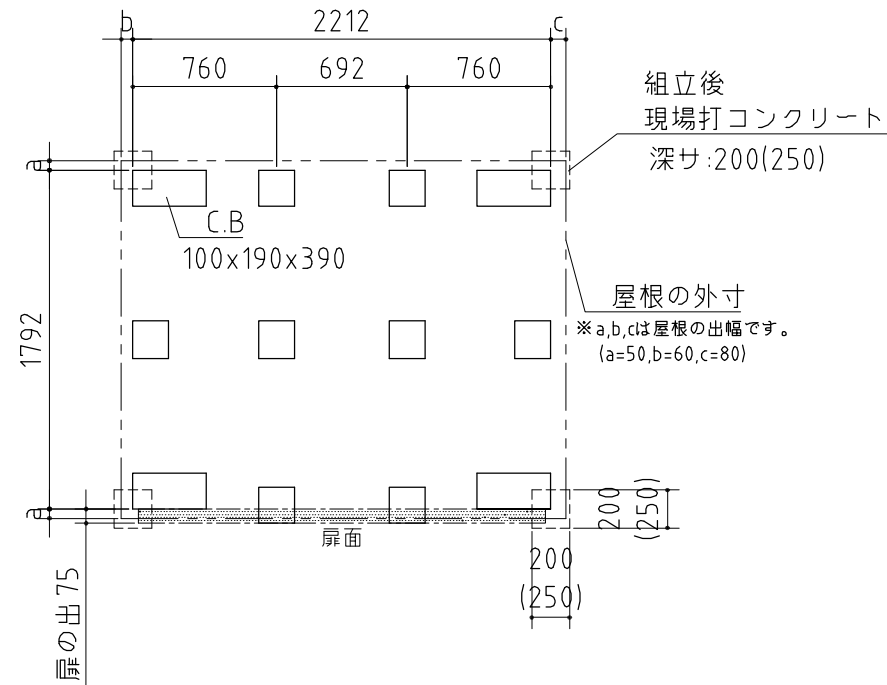
( )内寸法はNXN-40HB用
