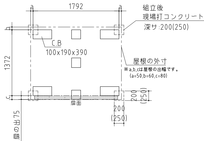
( )内寸法はNXN-25HA用
