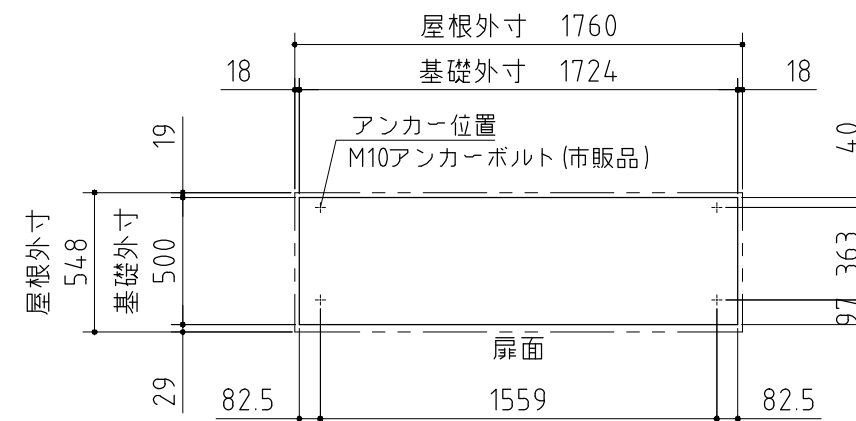
ベタ基礎図
