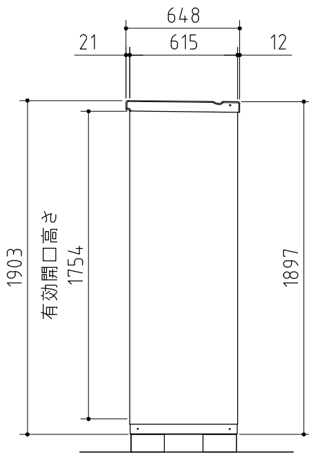
側面図
