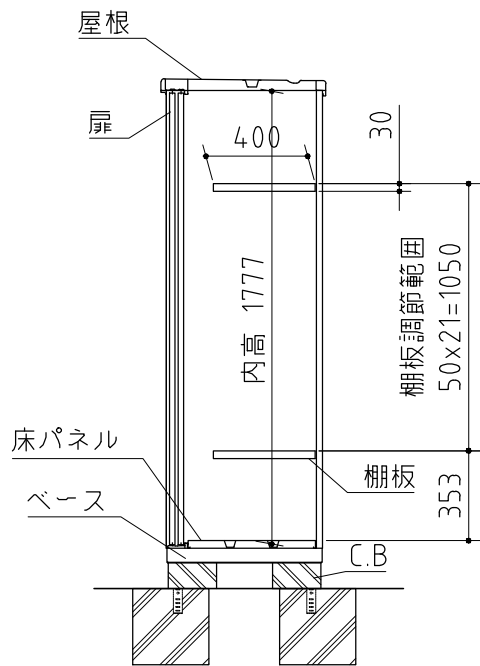
断面図
