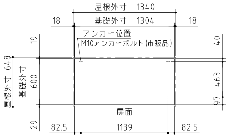
ベタ基礎図
