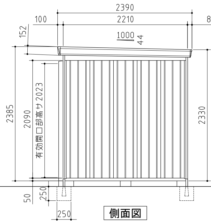
外形図
