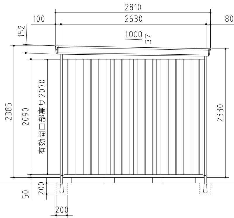
側面図
