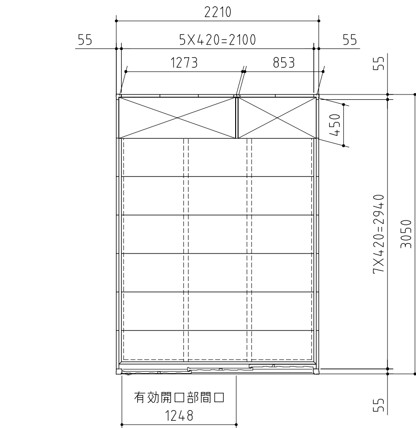
平面図
