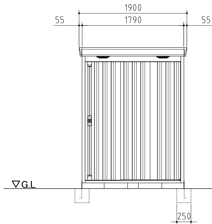
正面図
