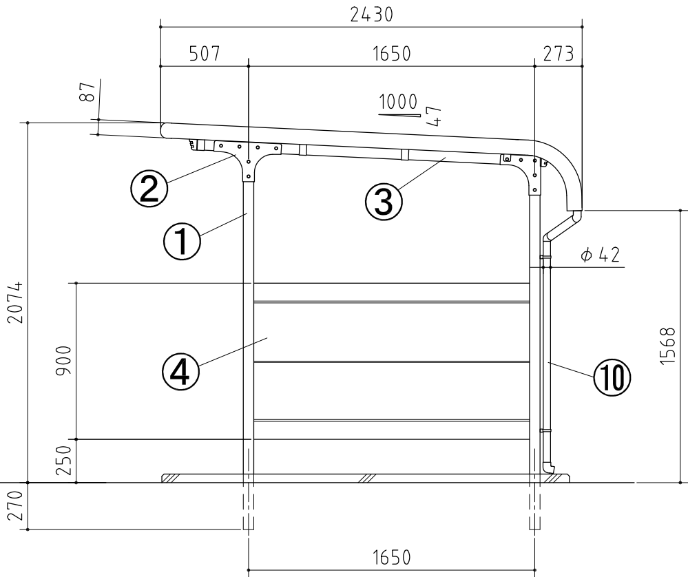
側面図
