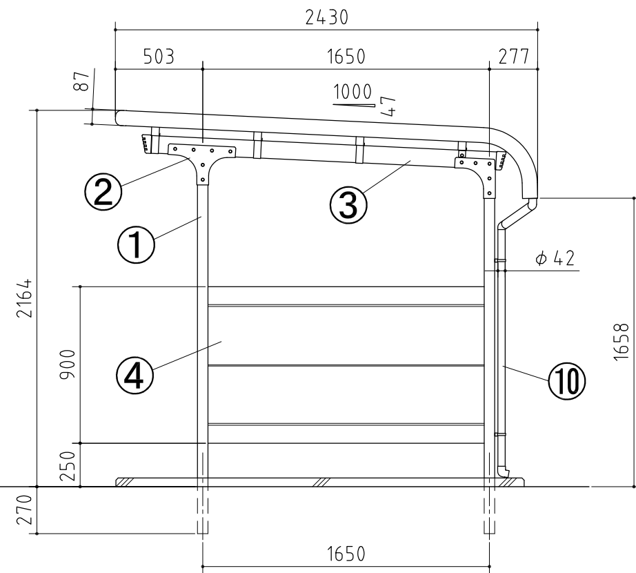
側面図
