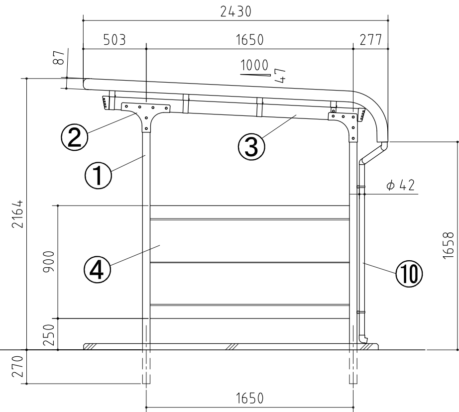
側面図
