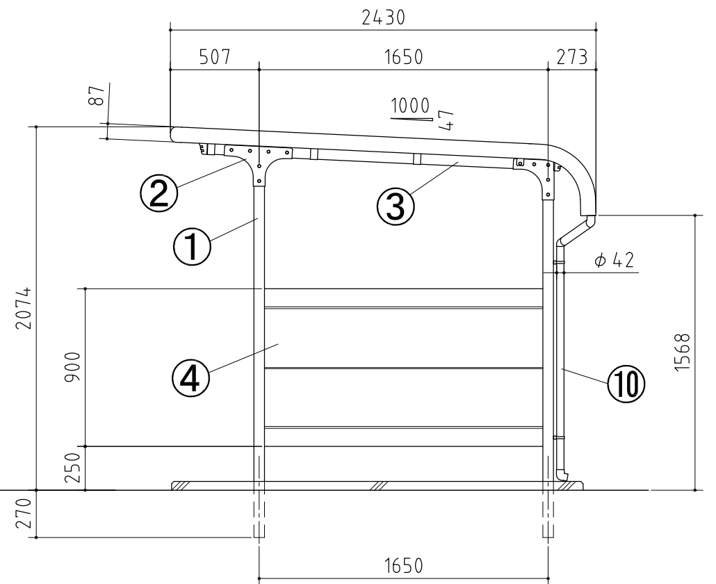
側面図
