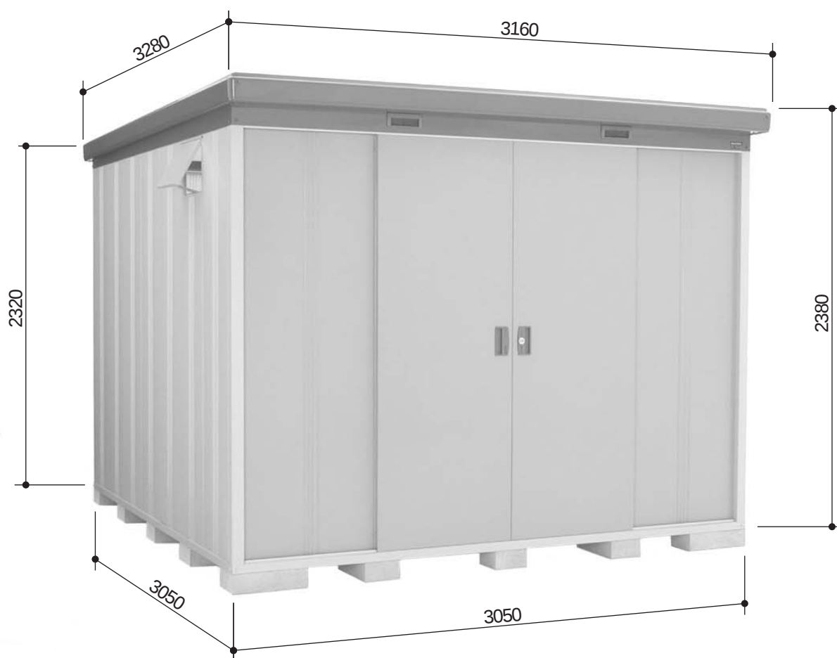
MBW -95FH型 寸法図
