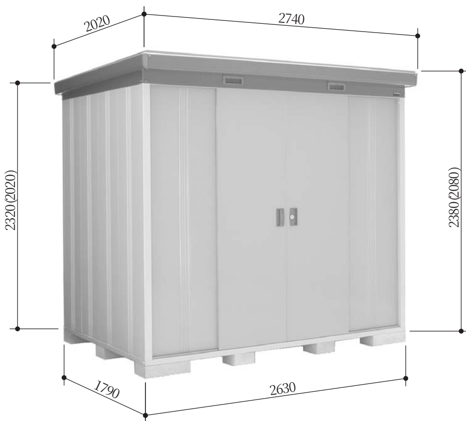
MBW -50・50H型 寸法図 (写真は、MBW -50H型です)
