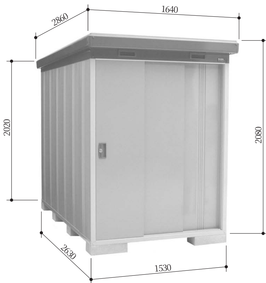
MBW-41型 寸法図
