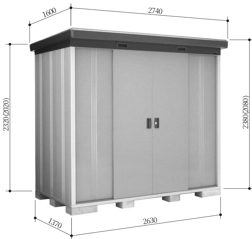
MBW -36・36H型 寸法図 (写真は、MBW -36H型です)
