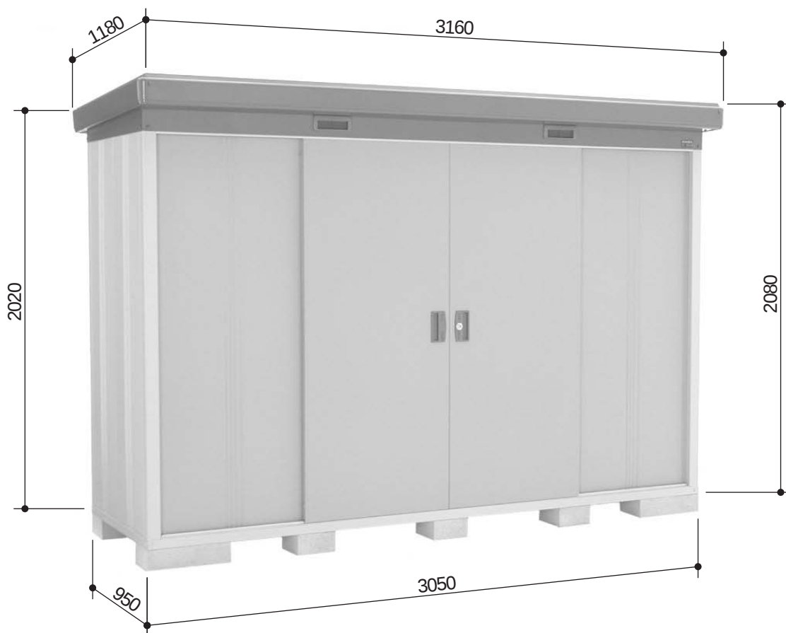
M BW -30F型 寸法図
