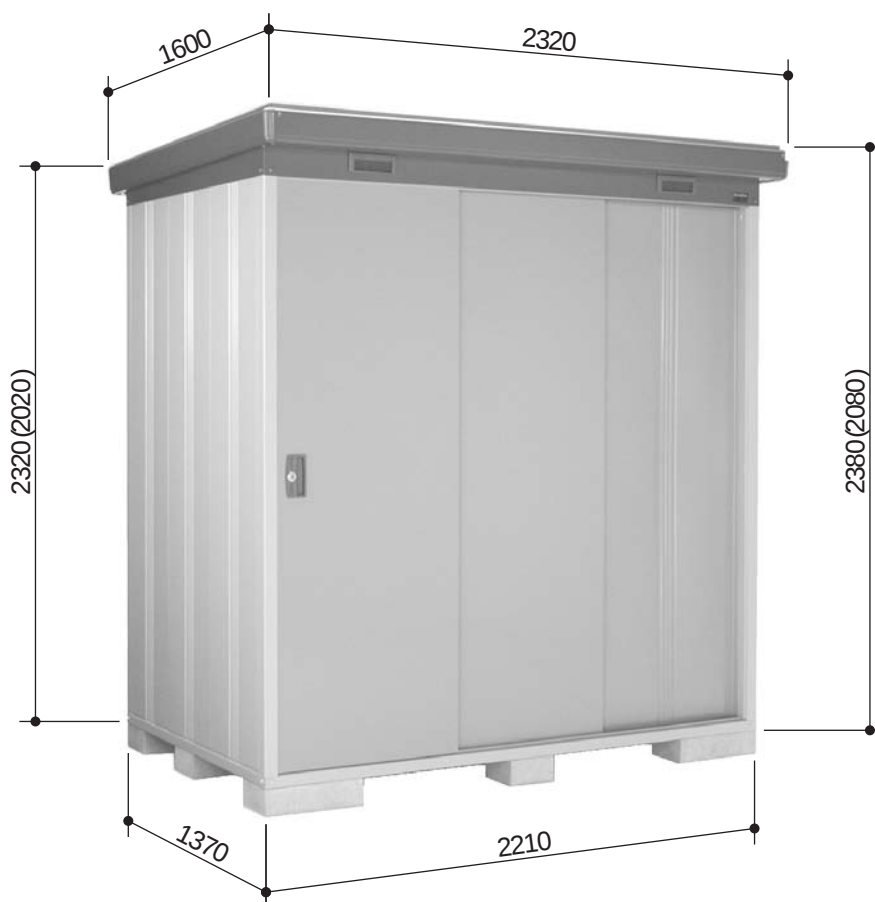
MBW -30・30H型 寸法図 (写真は、MBW -30H型です。)
