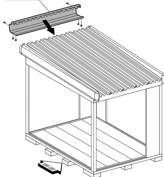
(25)鼻隠し前
