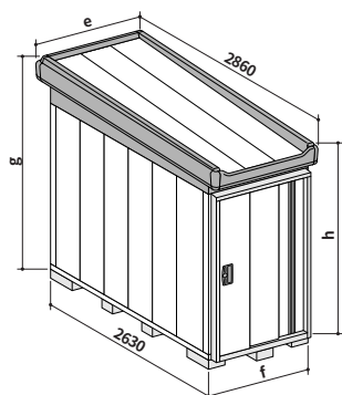
CA・CHA型 寸法図 (単位: mm)
