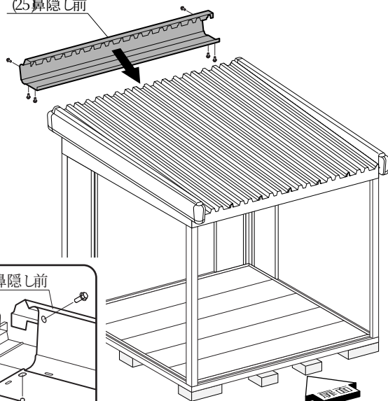
(25)鼻隠し前
