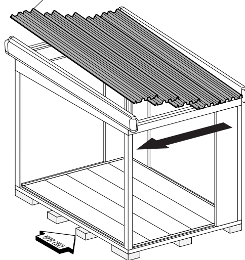
(24)屋根パネル
