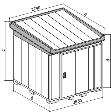
A型 寸法図 (単位: mm)
