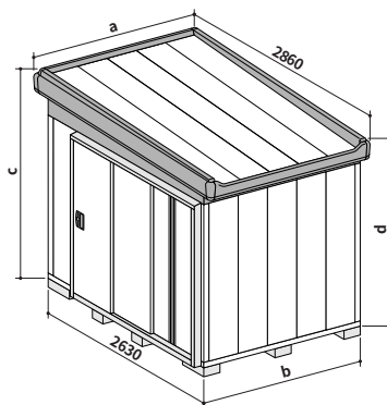
B型 寸法図 (単位: mm)
