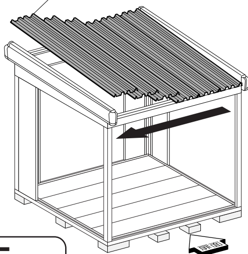
(24)屋根パネル
