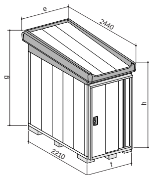
CA・CHA型 寸法図 (単位: mm) イラストは、MBW -30CA型です。 機種ごとの寸法は、下表を参考にしてください。
