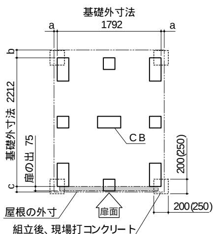
MBW -40CA MBW -40CHA (内寸法はMBW-40CHA用です。)
