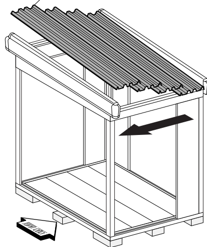
(24)屋根パネル
