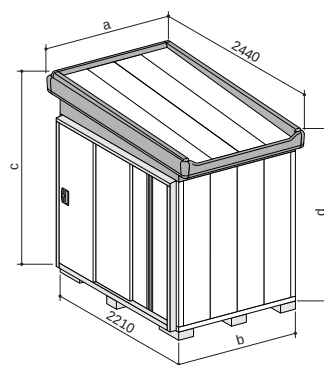
B型 寸法図 (単位: mm) イラストは、MBW -40B型です。 機種ごとの寸法は、下表を参考にしてください。
