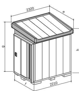
CB・CHB型 寸法図 (単位: mm) イラストは、MBW -30CB型です。 機種ごとの寸法は、下表を参考にしてください。
