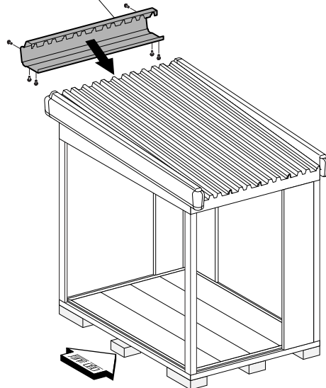
(25)鼻隠し前
