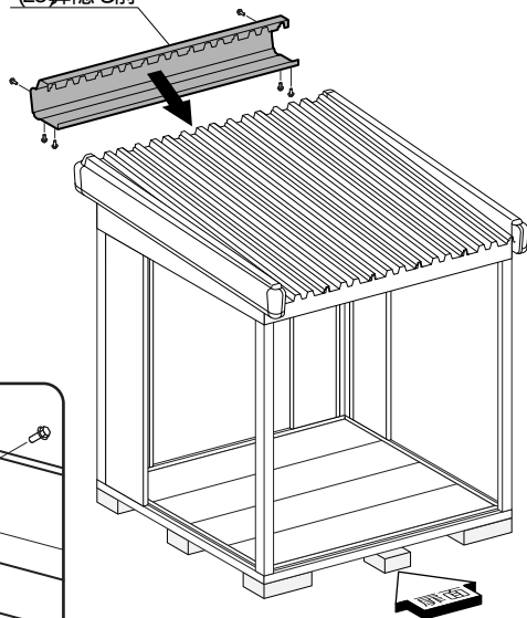
(25)鼻隠し前
