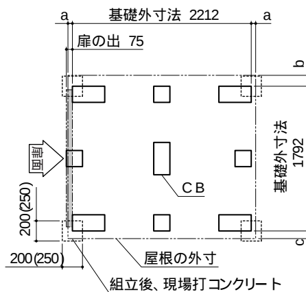
MBW -40CB MBW -40CHB ( 内寸法はMBW-40CHB用です。)
