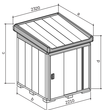
A型 寸法図 (単位: mm) イラストは、MBW -40A型です。 機種ごとの寸法は、下表を参考にしてください。
