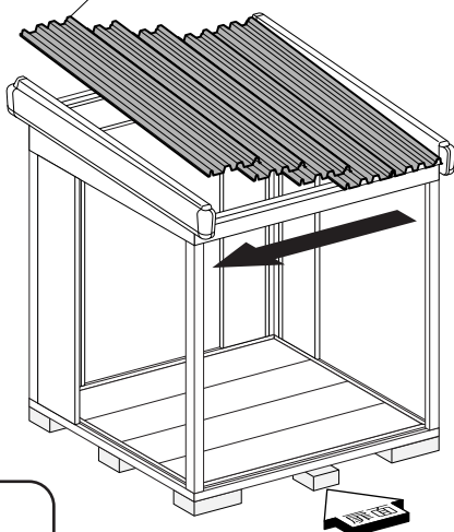
(24)屋根パネル
