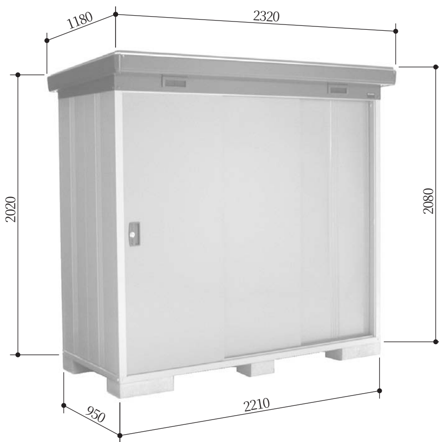
MBW -21型 寸法図
