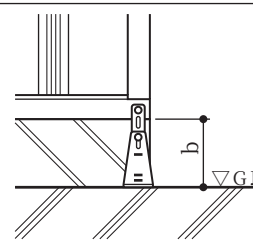
地盤がコンクリートの場合
