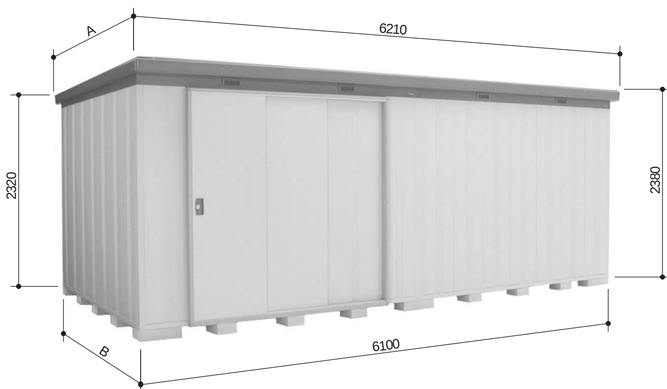
MBW -136H・162H・188H・215H型 寸法図 (写真は、MBW -188H型です。)
