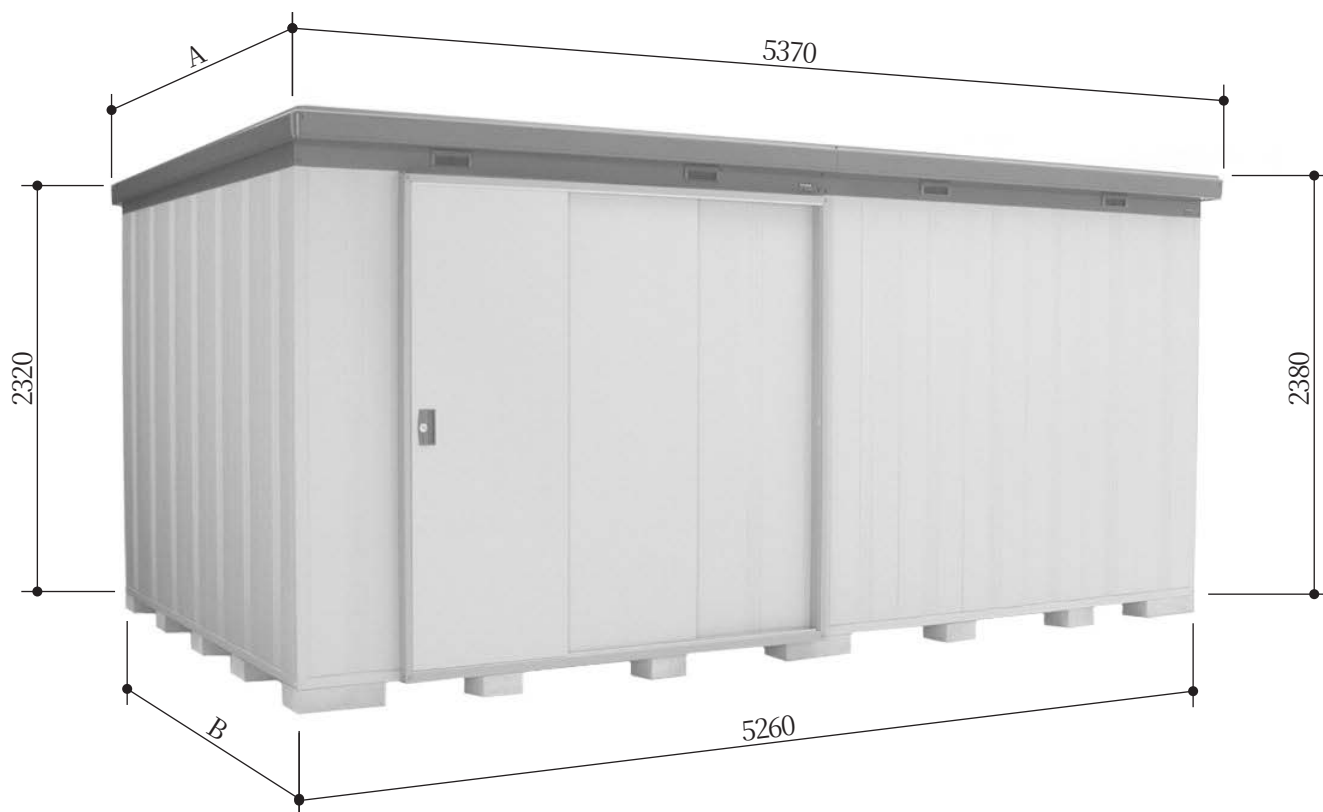
MBW -100H・120H・140H・160H・185H型 寸法図 (写真は、MBW -160H型です。)
