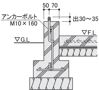
A—A' 断面
