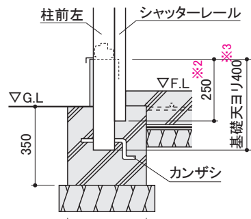
B-B' 断面
