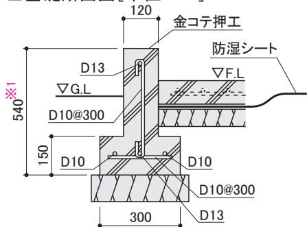
■基礎断面図[単位:mm]
