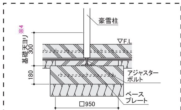
E-E' 断面（豪雪地型・耐力壁設置箇所のみ）
