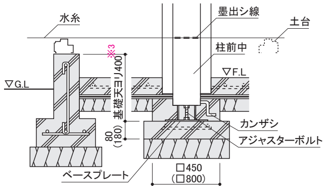
D-D' 断面
