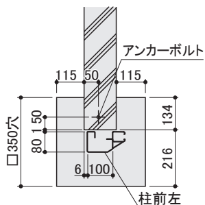
C部
