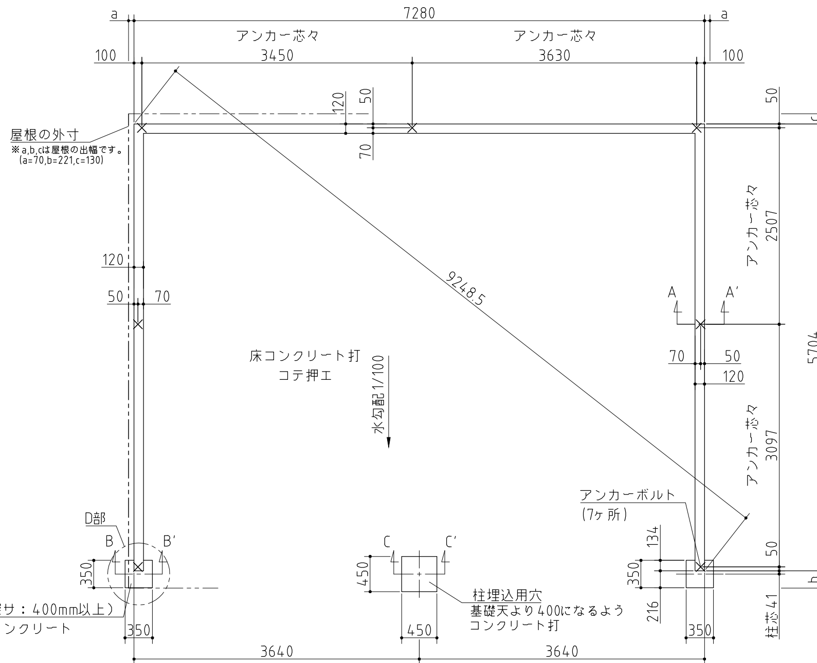
基礎詳細図 S=1/20
