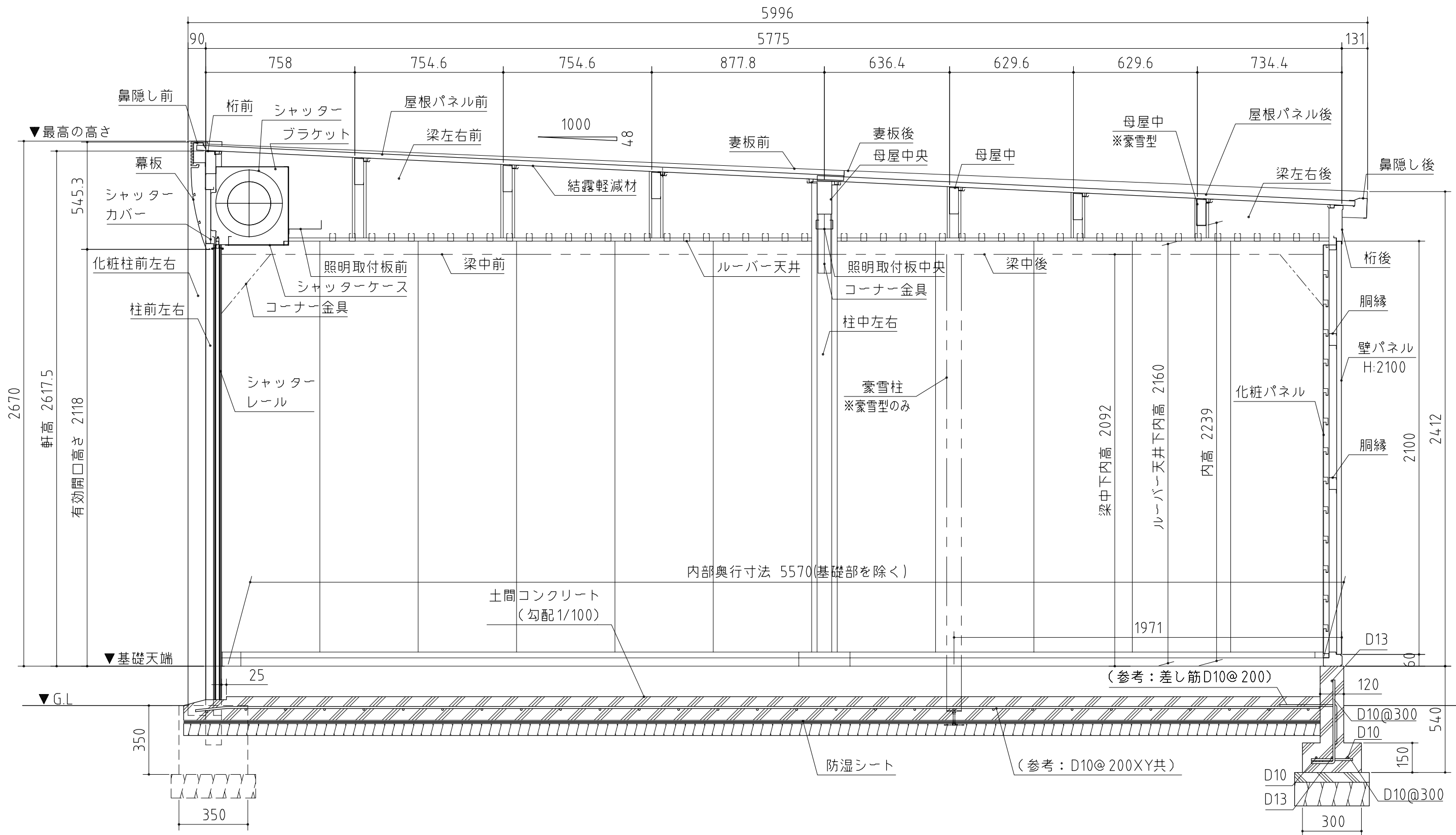
断面図(側面) <縮尺> S=1/20 ~一般型・豪雪型~ 機種名 DR-3157・3657HPB・HYB 3157・3657HPB・HYB-N[連棟数]
