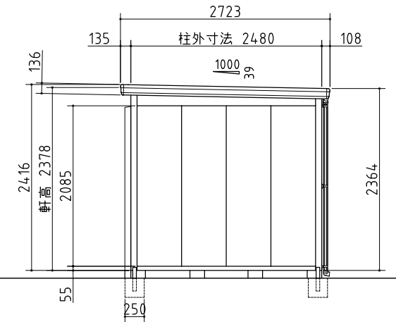
右側面図
