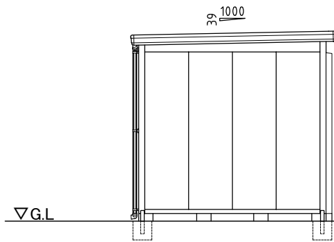
左側面図
