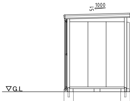
左側面図
