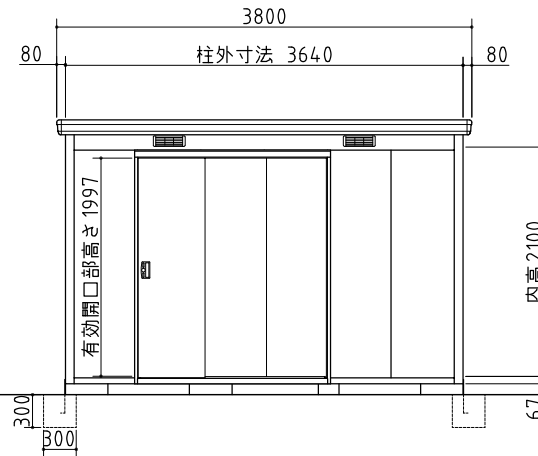
正面図
