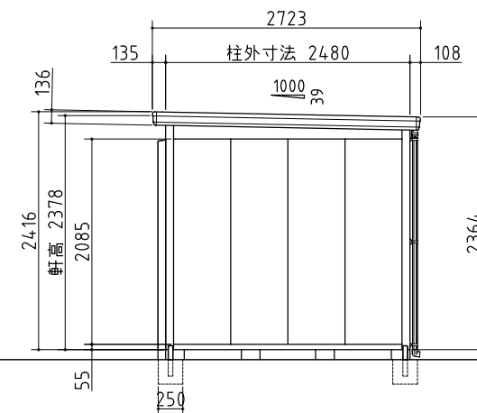
右側面図
