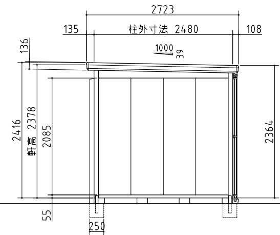
右側面図
