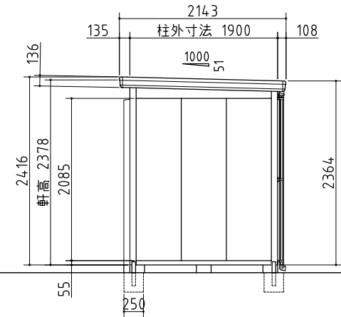
右側面図
