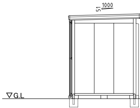
左側面図
