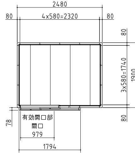
平面図
