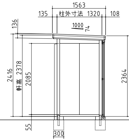
右側面図
