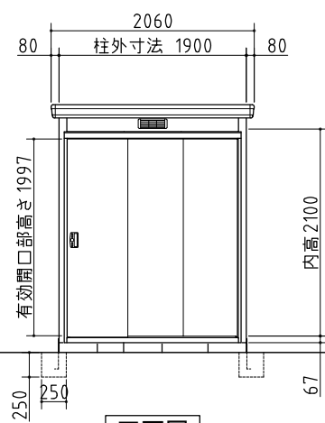
正面図
