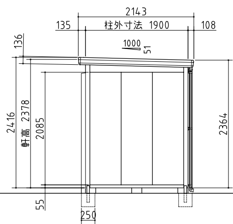
右側面図
