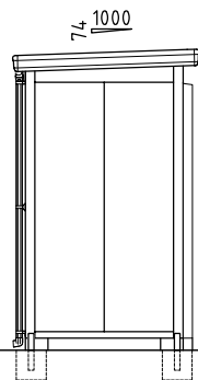
左側面図
