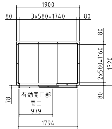
平面図
