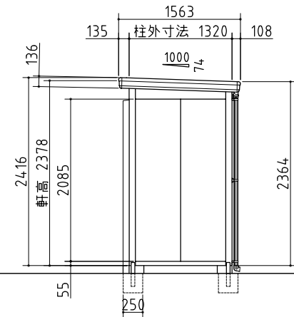
右側面図
