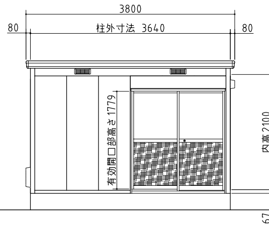
正面図
