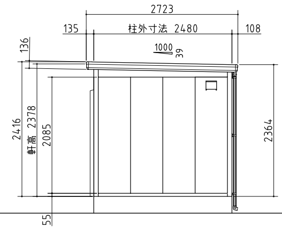
右側面図
