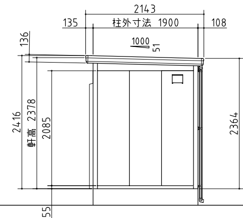
右側面図
