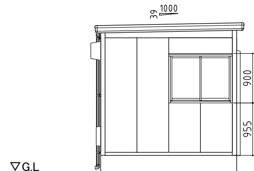
左側面図
