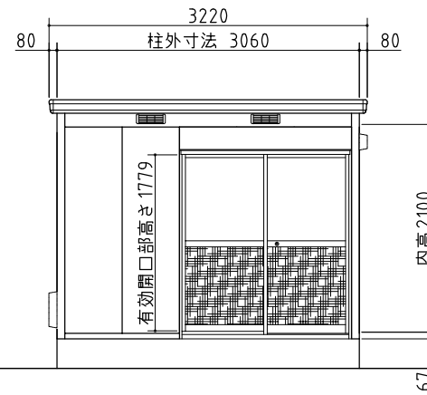
正面図
