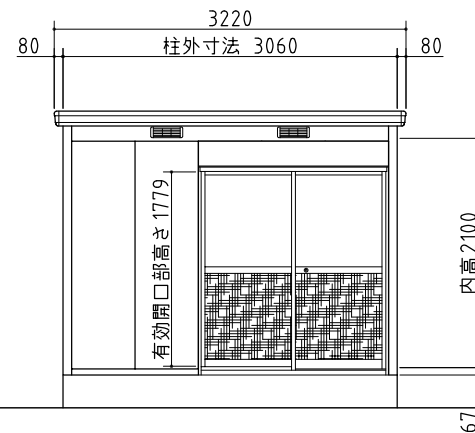
正面図
