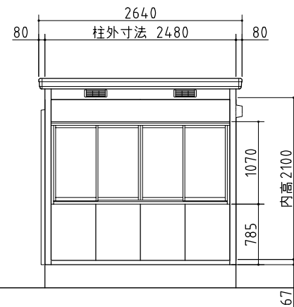
正面図
