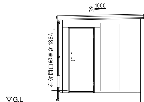
左側面図
