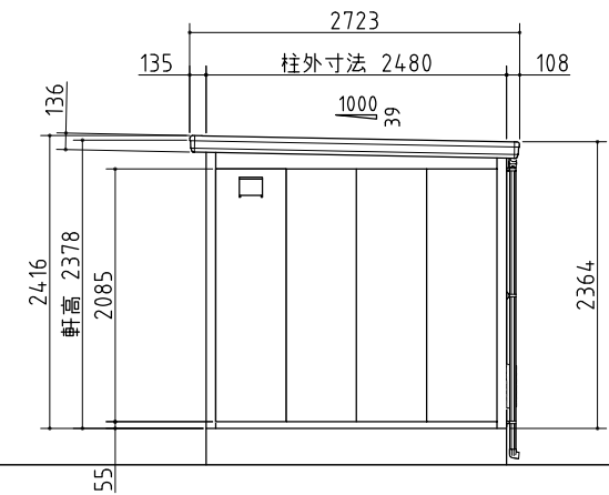
右側面図
