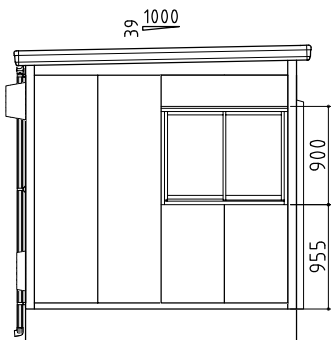
左側面図
